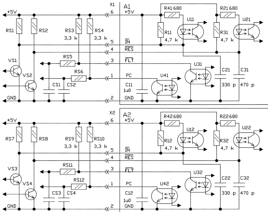
Рисунок 2 - Вариант подключения драйвера
