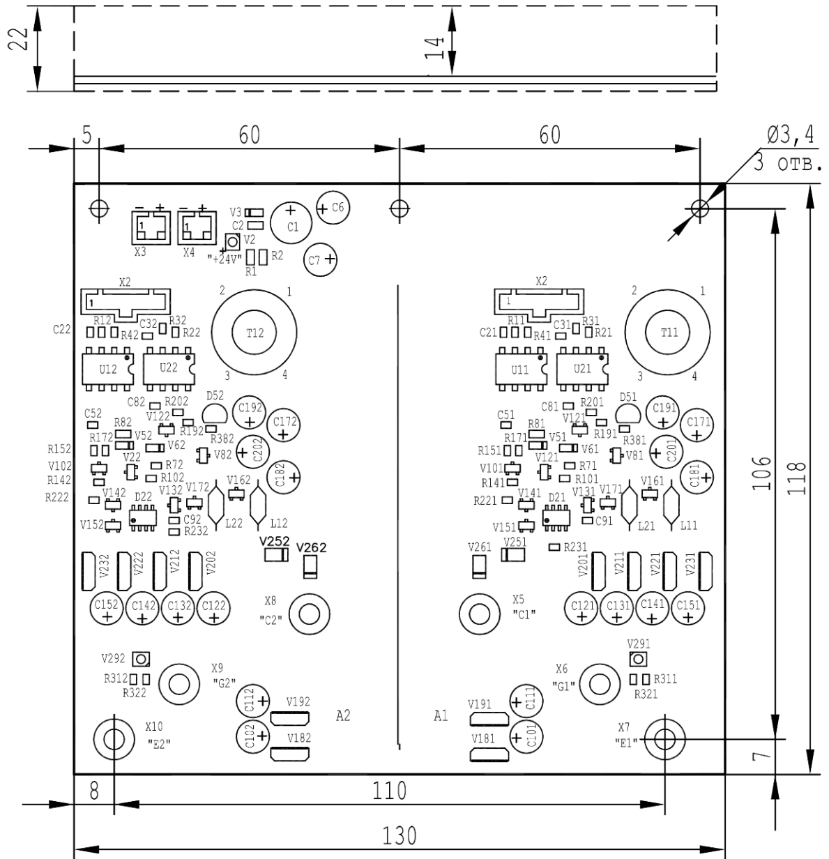
Рисунок 1 – Габаритные и установочные размеры платы драйвера ДРИ21 -20-17-2ОП1Н-1
