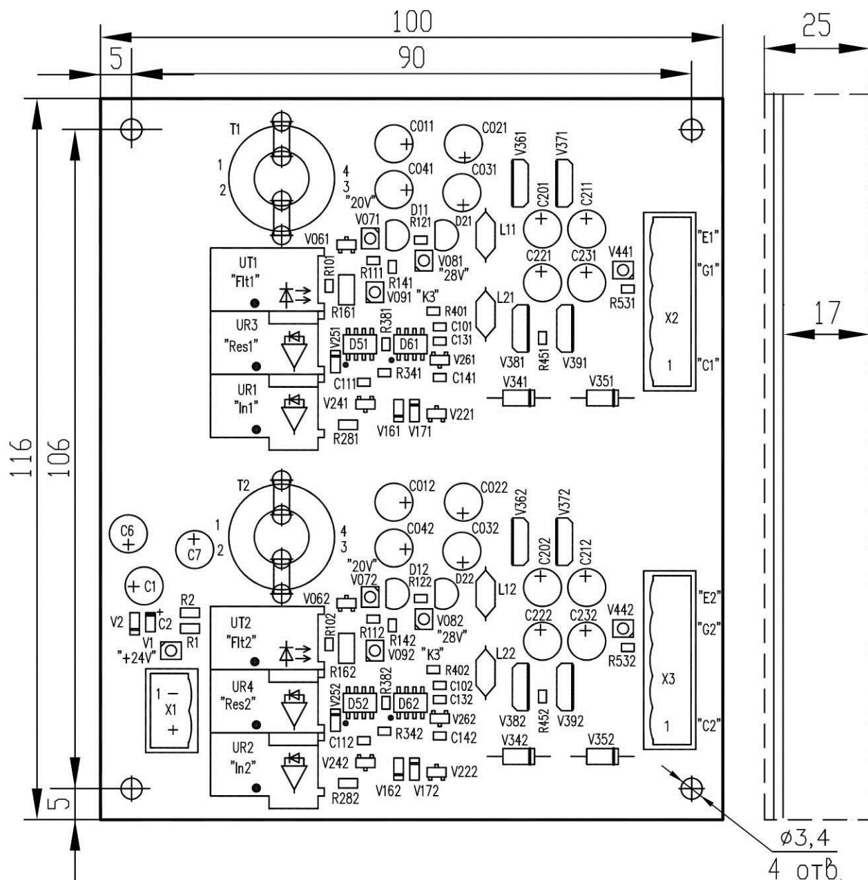
Рисунок 1 – Габаритные и установочные размеры платы драйвера ДРИ21 -10-17-3ФП1К-3
