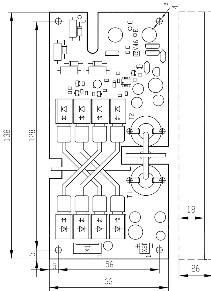
Рисунок 1 – Габаритные и установочные размеры платы драйвера ДРИ11 -10-33.6ОП1К-1
